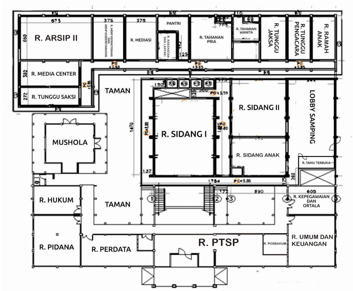
Denah Lantai 1 Kantor Pengadilan Negeri Banyumas Kelas II.
