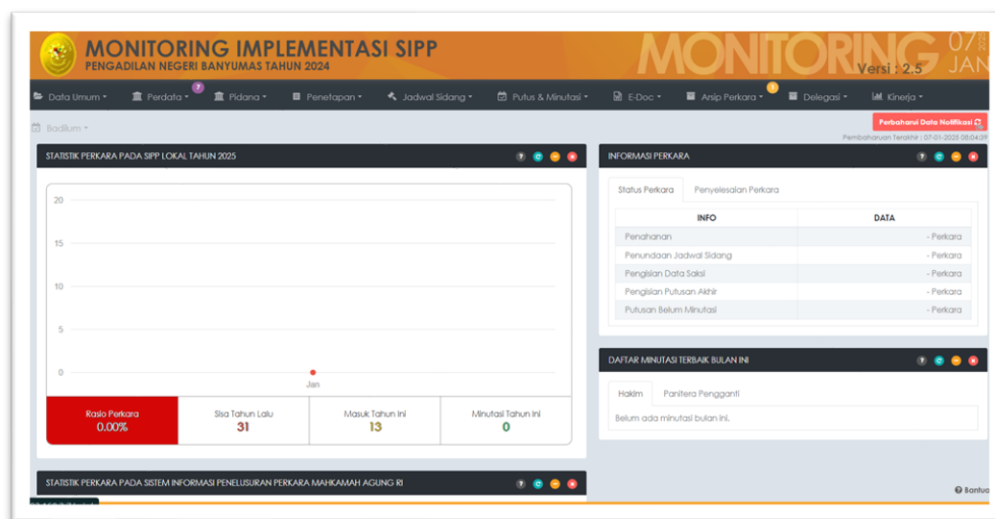
Gambar 4.4 Implementasi MIS
